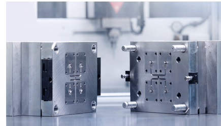
Metallpulverspritzgusswerkzeug mit 4 Kavitäten
