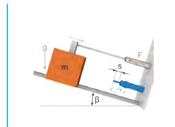
L10.利用驱动力在斜面上向下运动的质量
