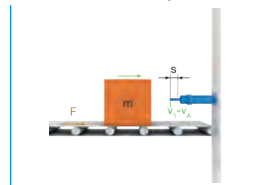
L7. Masa desplazada horizontalmente con fuerza motriz accionada por fricción
