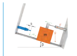
L11. Masa desplazada hacia arriba con fuerza motriz en un plano inclinado
