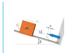
L9. Masa desplazada hacia abajo con fuerza motriz opuesta en un plano inclinado
