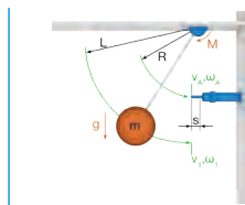
R2. Masa oscilante hacia abajo con par opuesto a) con impacto horizontal
