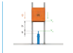
L2. Masa desplazada hacia abajo con fuerza motriz opuesta
