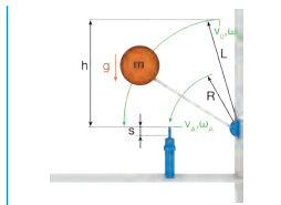
R1. Masa de oscilación libre b) con impacto vertical
