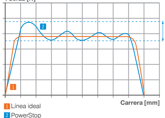
Fuerza [N]
