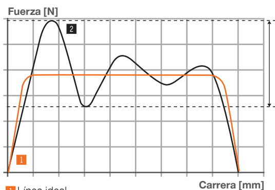
1 Línea ideal 2 Amortiguador convencional
