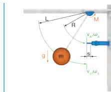
R3. Masa oscilante hacia abajo con par a) con impacto horizontal
