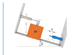
L10. Masa desplazada hacia abajo con fuerza motriz en un plano inclinado
