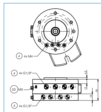
Paso de aire sin tubos (en el lado de la herramienta)
