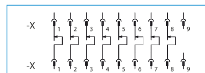
Disposición de los pines
